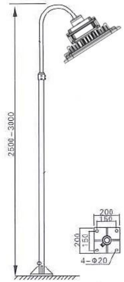
G. Pole Mount
